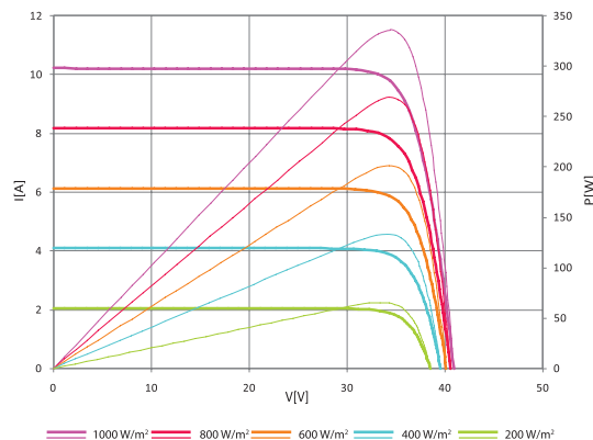
CHARAKTERYSTYKA PRĄDOWO-NAPIĘCIOWA
