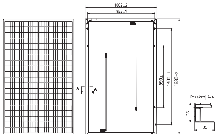
WYMIARY MODUŁU
