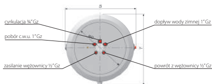
NIBE BA-WH 8040/8050/XX-2F
