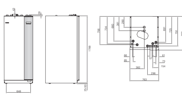
NIBE VVM 500
