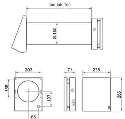
NIBE DVC 10
