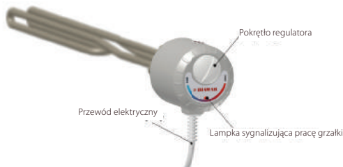
Budowa modułów grzejnych ME 0015-ME 0030
