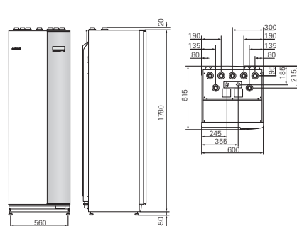
NIBE VVM 310/320
