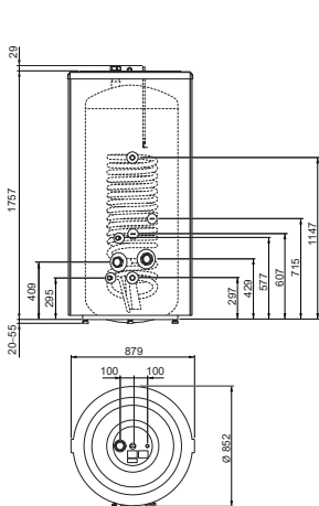
NIBE VPB 500
