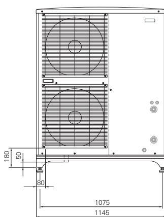
NIBE F2040-16
