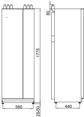
NIBE VPB 300 / VPBS 300
