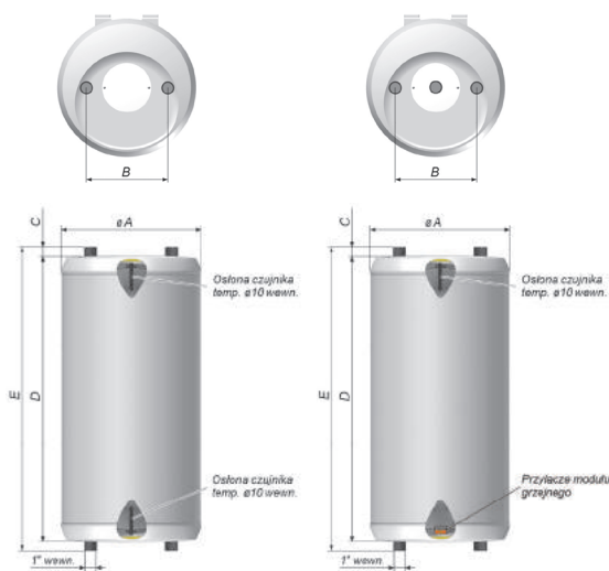
NIBE UKV 100
