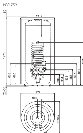
NIBE VPB 750
