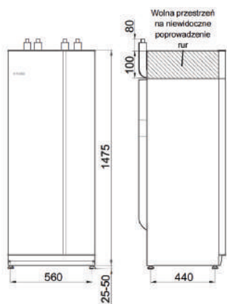
NIBE VPB 200
