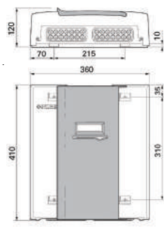
NIBE SMO 40
