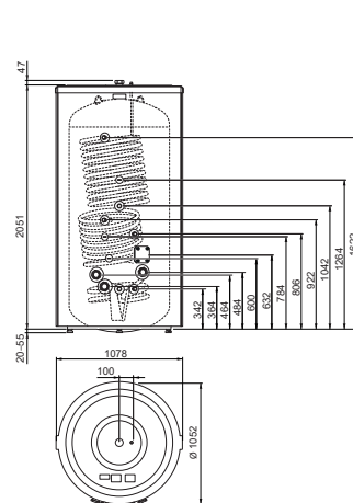
NIBE VPB 1000
