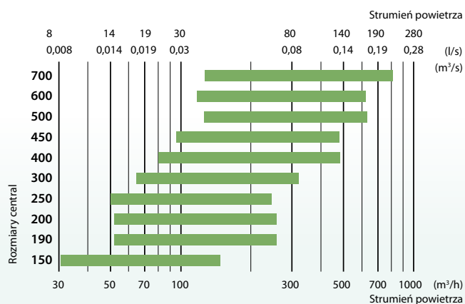
Rozmiary i wydajność central Domekt R
